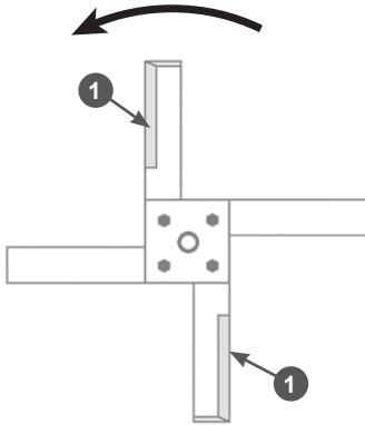
Рис. 4 Правильная установка фрез
