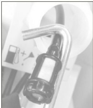
Рис. 14 Извлечение топливного фильтра
