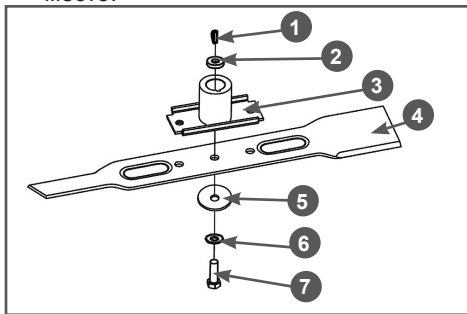
Рис. 23 Установка ножа
