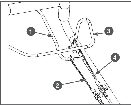
Рис. 6 Правильная установка тросов
