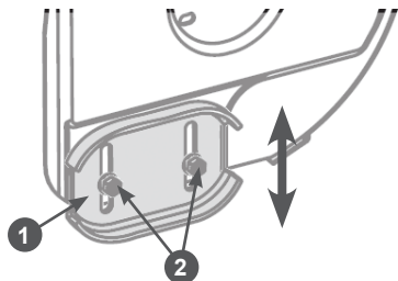
Рис. 29 Регулировка высоты забора снега 1. Ползок 2. Гайка (2 шт.)
