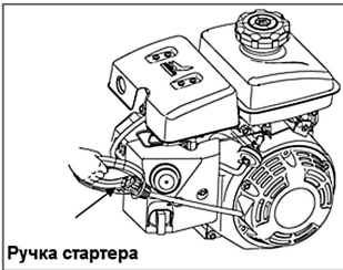
Рис. 9 Запуск двигателя
