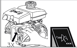
Рис.8 Ручной топливный насос
