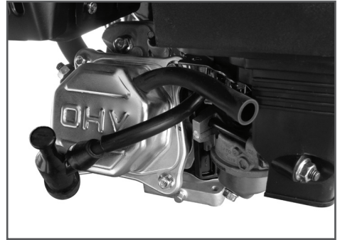
Рис. 8 Трубка сапуна
