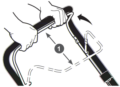
Рис. 12 Рычаг остановки двигателя
