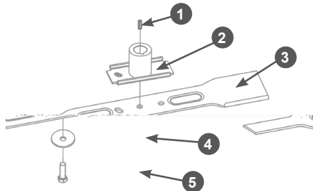
Рис. 23 Установка ножа
