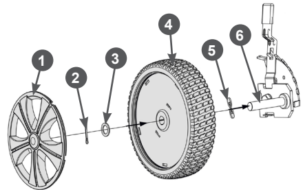
Рис. 3 Схема установки колёс
