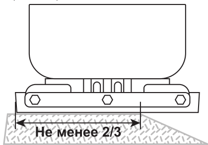
Рис. 14 Расположение виброплиты на краю обрабатываемой поверхности
