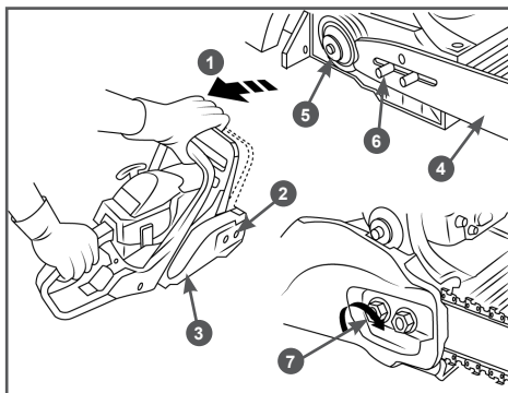
Рис. 2 Установка шины
