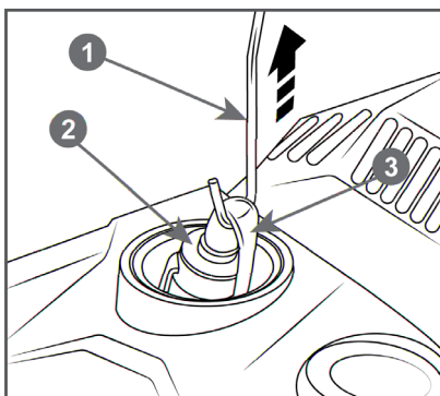
Рис. 22 Обслуживание топливного фильтра
