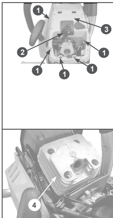
Рис. 23 Очистка охлаждающих ребер цилиндра
