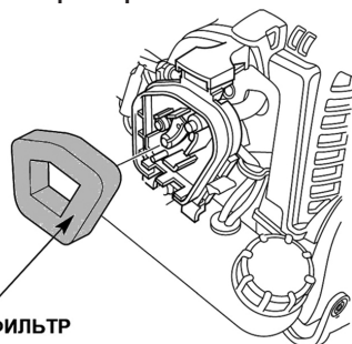
Рис. 17 Воздушный фильтр
