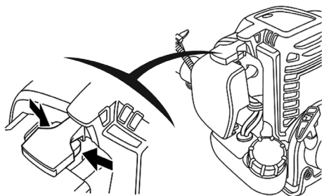
Рис. 16 Снятие крышки воздушного фильтра
