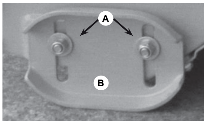
Рис.27 Регулировка высоты забора снега
