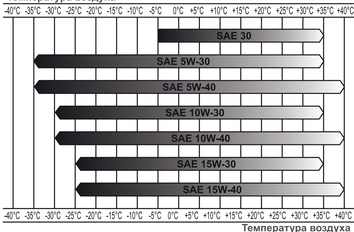
Рис.23 Таблица выбора моторного масла
