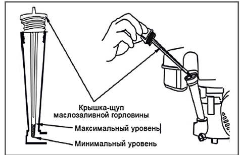
Рис.8 Проверка уровня масла в картере
