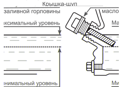
Рис. 6 Проверка уровня масла в картере
