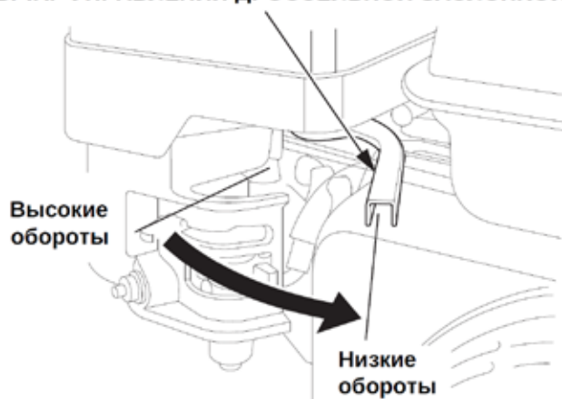
РЫЧАГ УПРАВЛЕНИЯ ДРОССЕЛЬНОЙ ЗАСЛОНКОЙ
