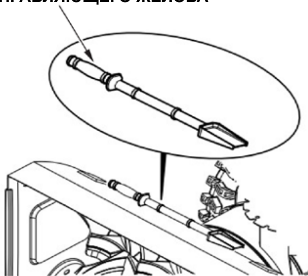
ЛОПАТКА ДЛЯ ПРОЧИСТКИ НАПРАВЛЯЮЩЕГО ЖЕЛОБА
