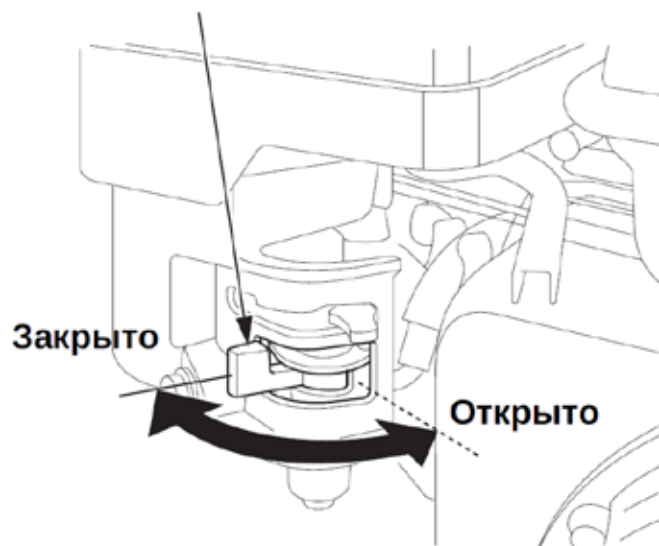
РЫЧАГ УПРАВЛЕНИЯ ТОПЛИВНЫМ КРАНОМ
