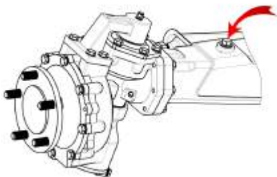
Рис. 10.1. Пробка заливная.
