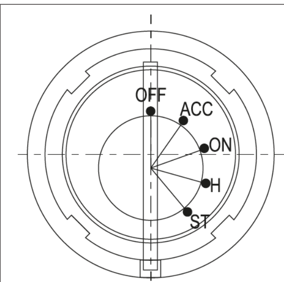
Рис. 9.1. Замок зажигания.
