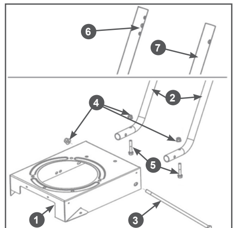
Рис. 2 Установка стоек рабочих рукояток
