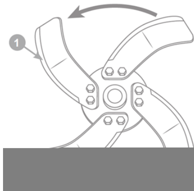
Рис. 4 Правильная установка фрез
