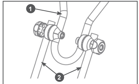
Рис. 7 Установка рабочих рукояток
